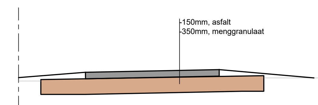
Doorsnede rijbaan Schaal 1:50
